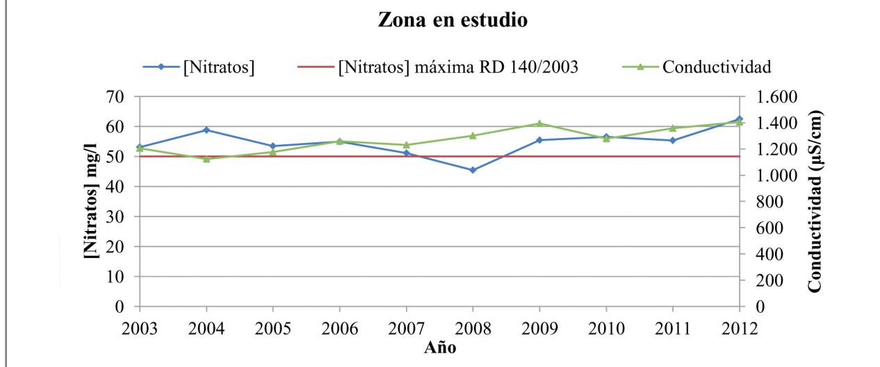
Figura 7. Relación entre la concentración de nitratos (mg/l) y la conductividad (µS/cm) en las aguas subterráneas de la zona en estudio.
